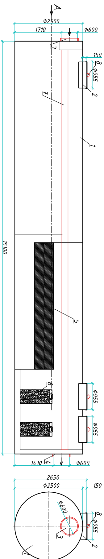
Разрез 1-1
